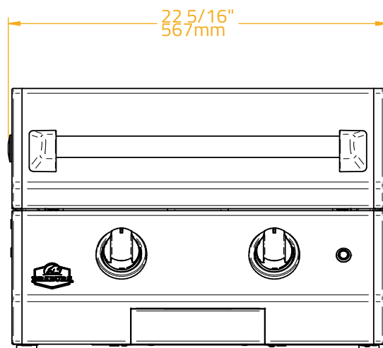
alzado
